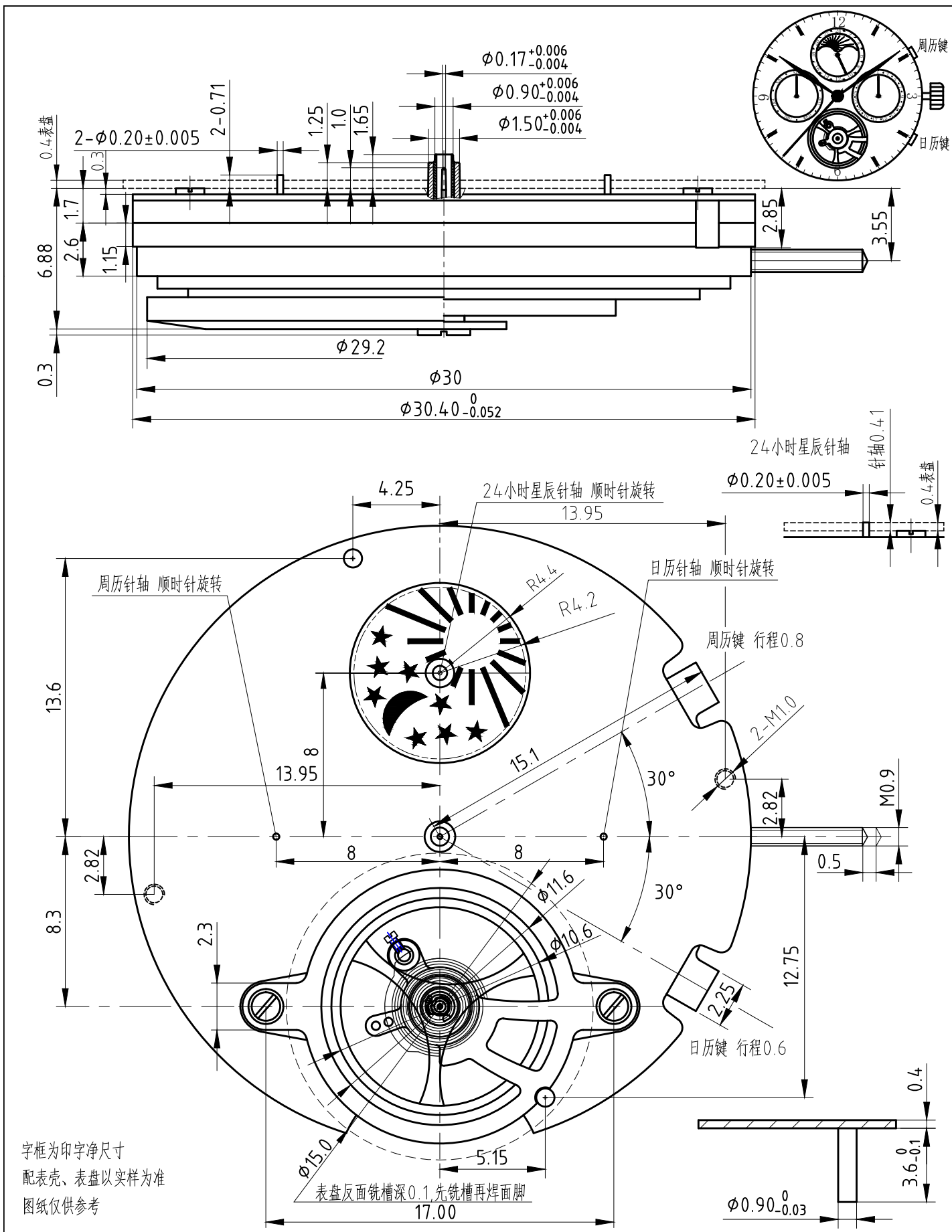
JH3022机芯外廓图
