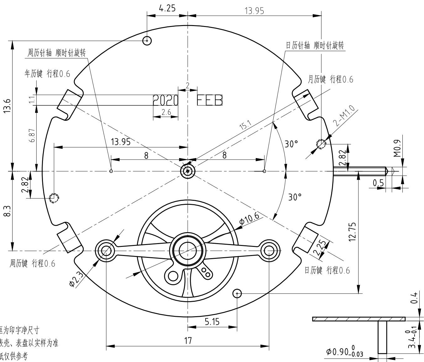
JH3005机芯外廓图
